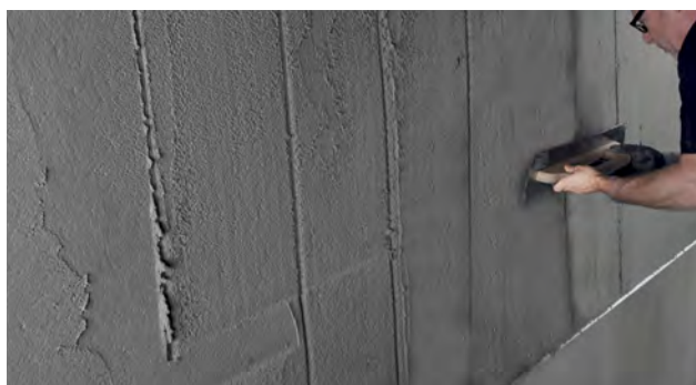
Påføring af Alfix DuraPuds 810 med stålbræt med afstandstænder
