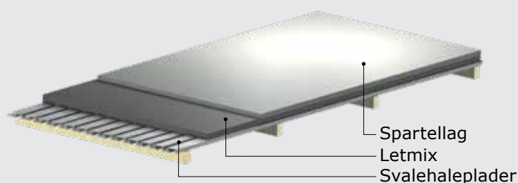
Støbning med PlaneMix 50 og 20 liter Leca (LetMix) på svalehaleplade
