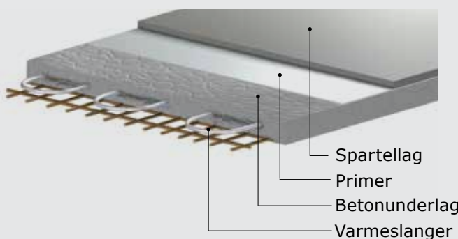
Spartling på betonunderlag med vandbårne varmeslanger
