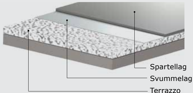
Spartling på eksisterende terrazzo
