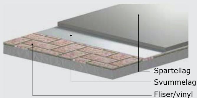
Spartling på eksisterende fliser/vinyl
