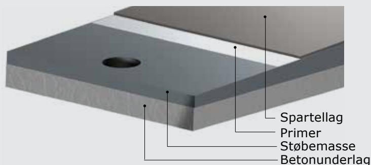
Eks. på fald mod afløb på mere end 2%
