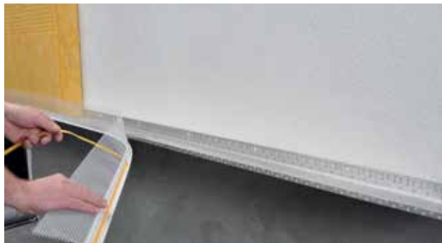
Montering av Alfix Bunnliste - Alu
