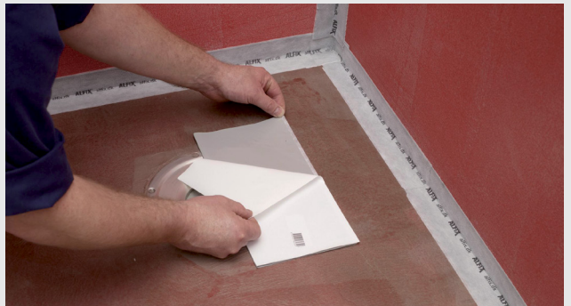
Montering av slukmansjett
