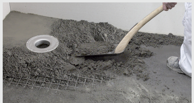
Oppbygging av fall med støpemasse
