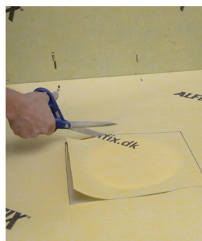
Alt. 1: Utskarning av folie vid brunnsmanschett
