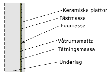
VT vägg (VTv och VTvF) (vertikalt snitt)
