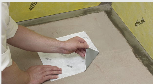
Montering av Alfix Brunnsmanschett
