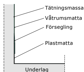
Anslutning mot plastmatta (vertikalt snitt)
